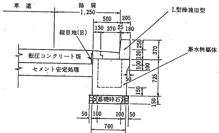
街渠枡(A)詳細図
