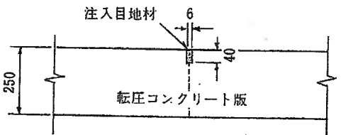
縦目地詳細図(A)
