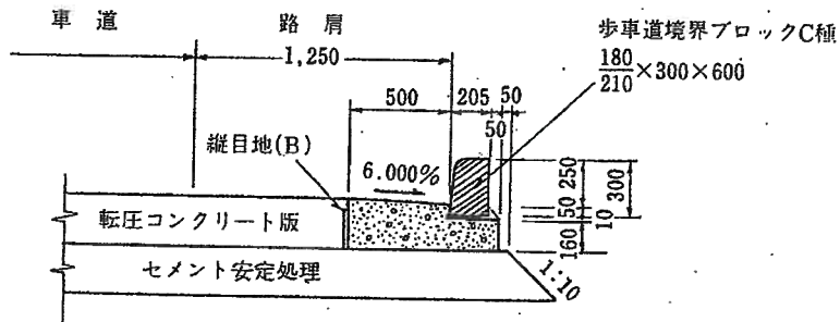
街渠(A)詳細図
