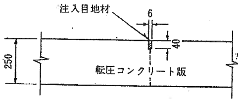
横収縮目地詳細図
