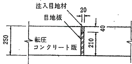
横膨張目地詳細図
